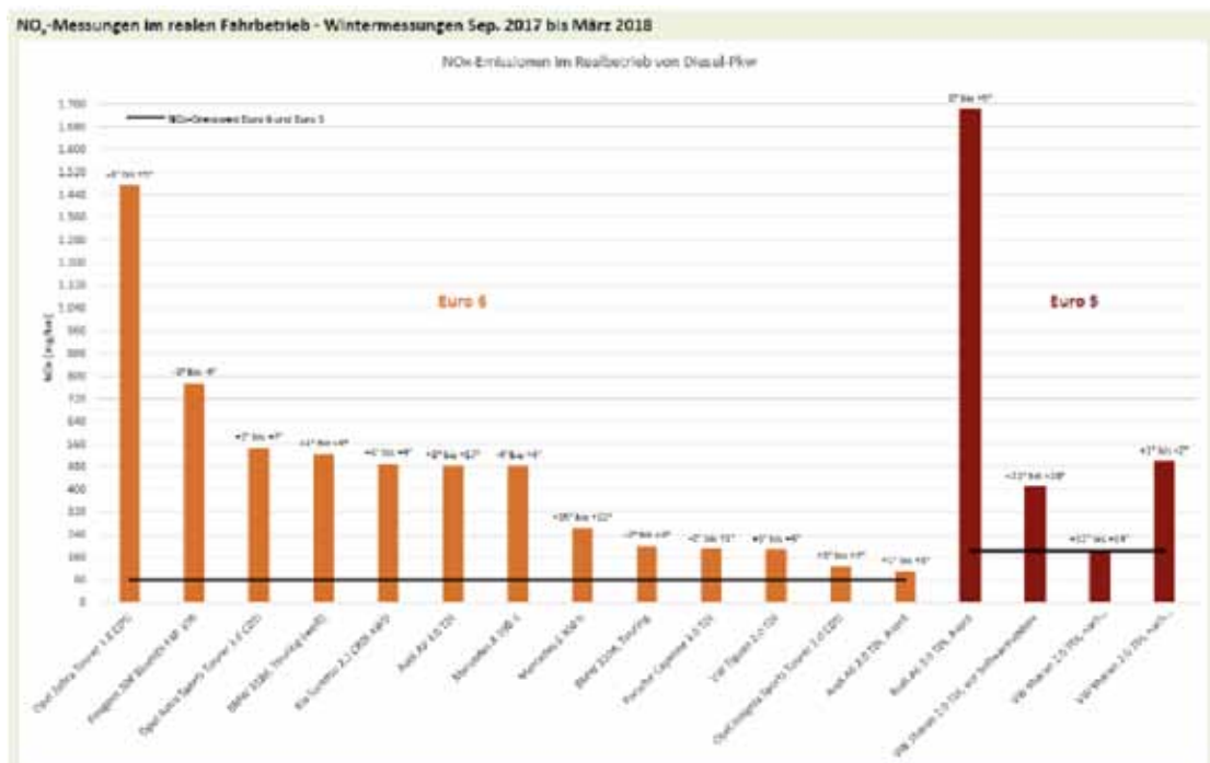
Abb. 6: Realemission NO x bei ausgewählten PKW im Winter- betrieb (DUH).
