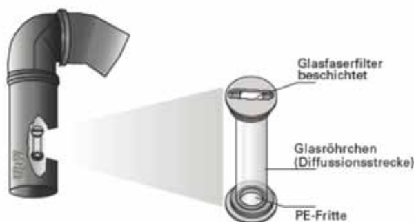
Abb.1: Aufbau der \text{NO}_2 -Messung mit Passiv- sammler
